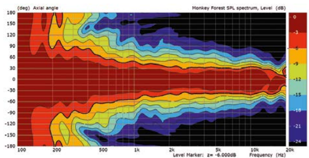
Horizontales Richtverhalten
