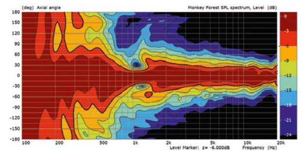
Vertikales Richtverhalten
