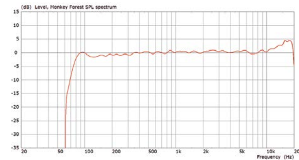
Frequenzgang (mit Controller)
