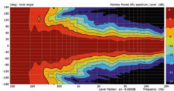
Horizontales Richtverhalten
