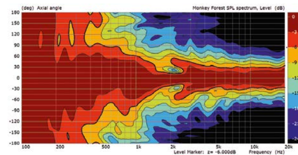
Vertikales Richtverhalten
