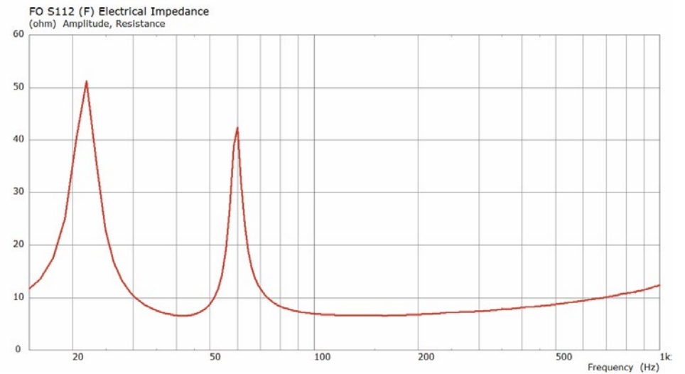
Elektrische Impedanz
