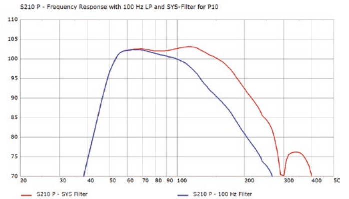
Frequenzgang SYS (rot) und 100 Hz (blau) (processed)
