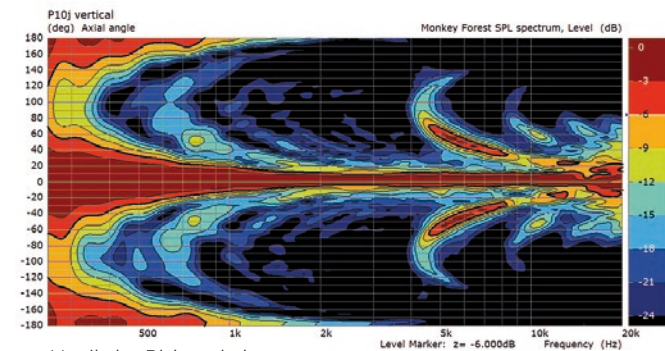
Vertikales Richtverhalten
