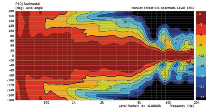
Horizontales Richtverhalten
