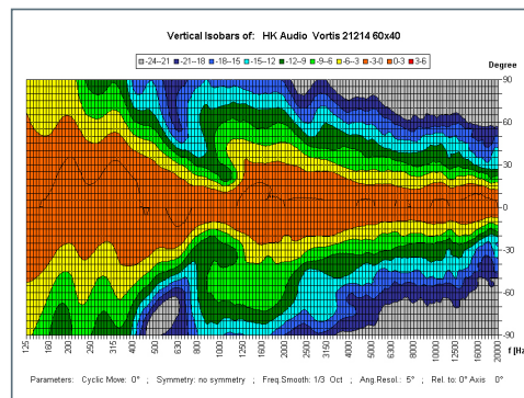
Hornvariante 60°x40° vertikal
