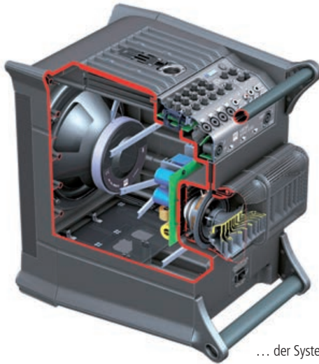
Im Querschnitt: Lucas „Nano 608i“ Top (rechts) und ...
